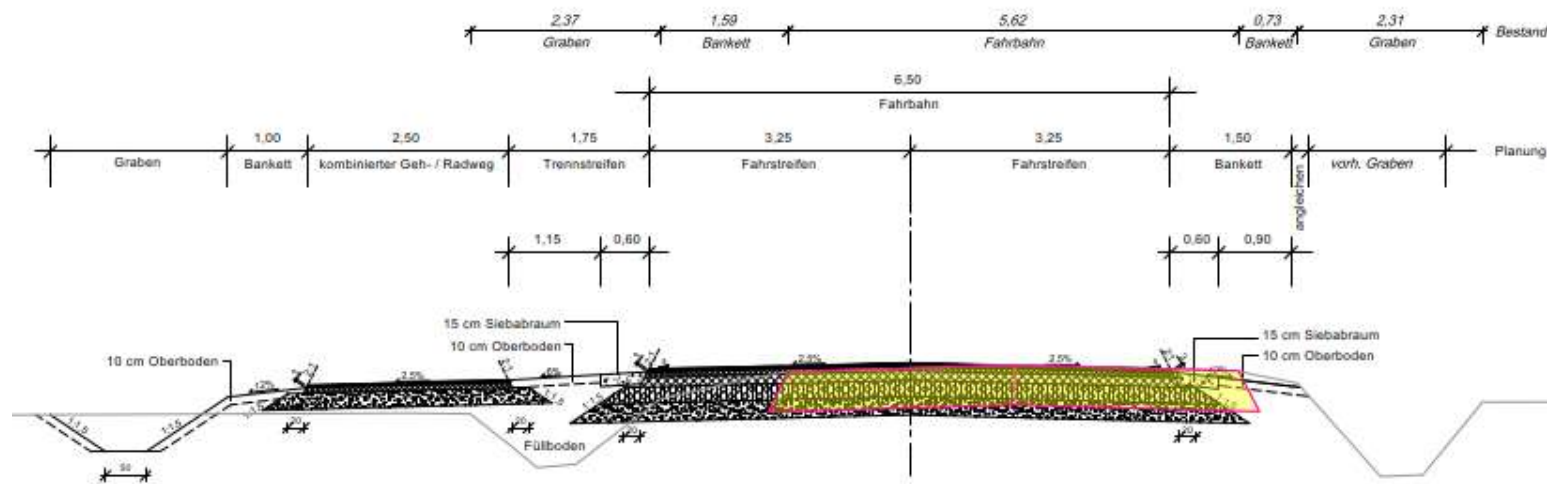
Deckenaufbau gem. RStO 12 Belastungsklasse 3,2, Tafel 1, Zeile 1
